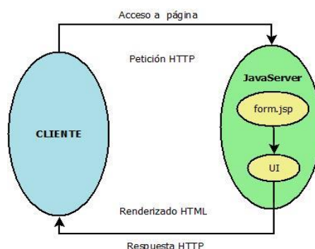
Ilustración 8 Diagrama de una aplicación JSF Fuente: Sandra Contento/Janneth Guamán
