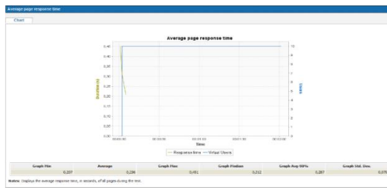
Ilustración 31 Tiempo promedio de Respuesta de Página – Primefaces y Richfaces Fuente: Sandra Contento/Janneth Guamán
