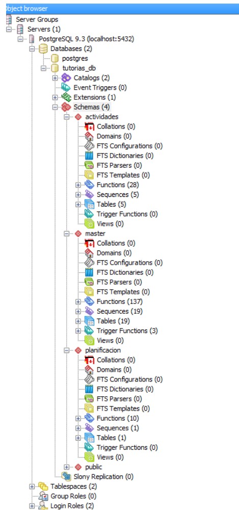
Ilustración 45 Esquema Base de Datos-Postgresql
