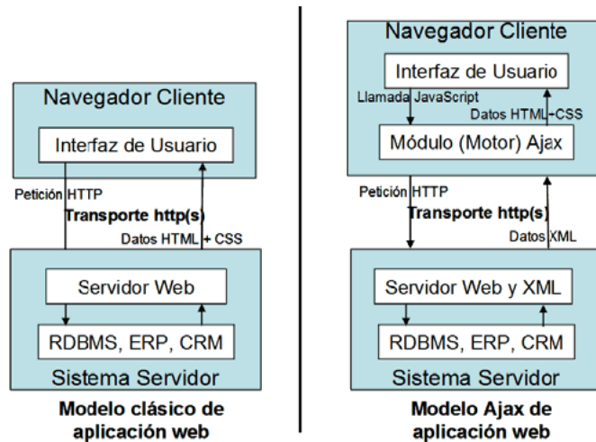
Ilustración 7 Modelo clásico de aplicación web y modelo AJAX de aplicación web Fuente: http://bit.ly/1H7uWWF
