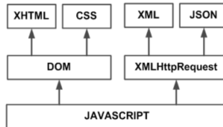
Ilustración 6 Tecnologías Agrupadas bajo el concepto de AJAX Fuente: http://librosweb.es/libro/ajax/capitulo_1.html
