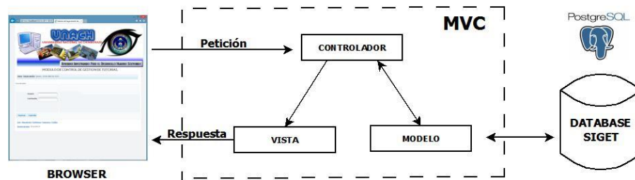
Ilustración 9 Modelo Vista Controlador
