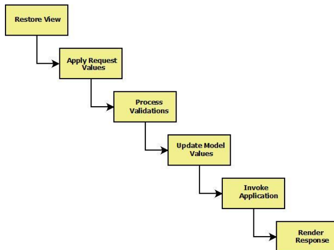
Ilustración 11 Ciclo de vida de Java Server Faces
