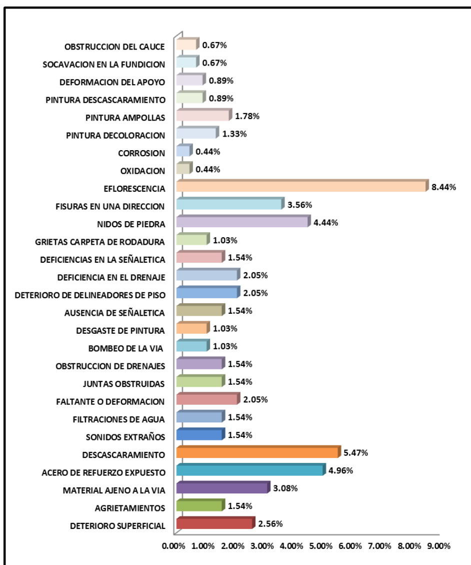
Figura No. 38: Patologías encontradas en el puente Cebadas Elaborado por: Henry Cain G y Marcelo Arcos.
