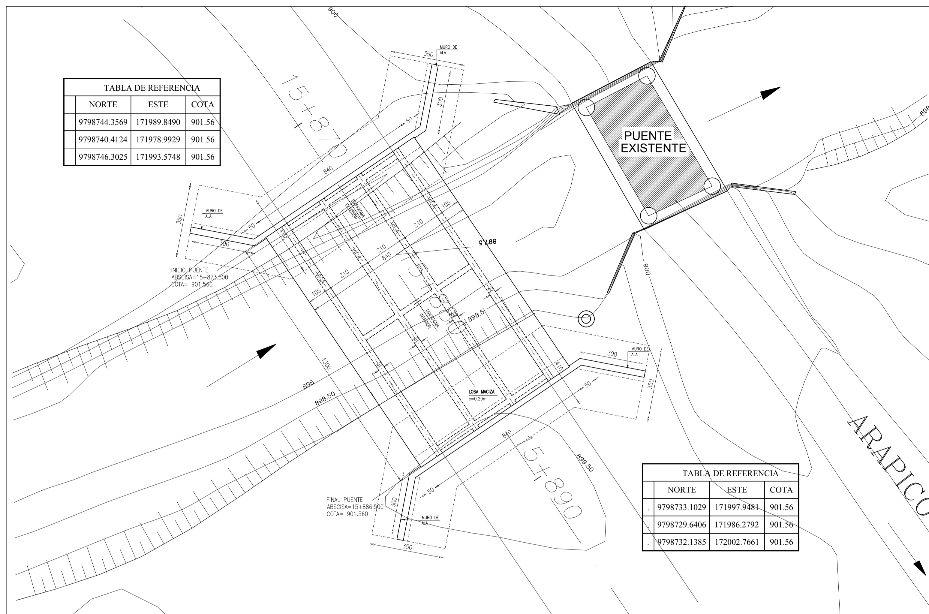
PUENTE SOBRE EL RIO RAMIREZ CORDERO. PLANTA ESC. 1:100
