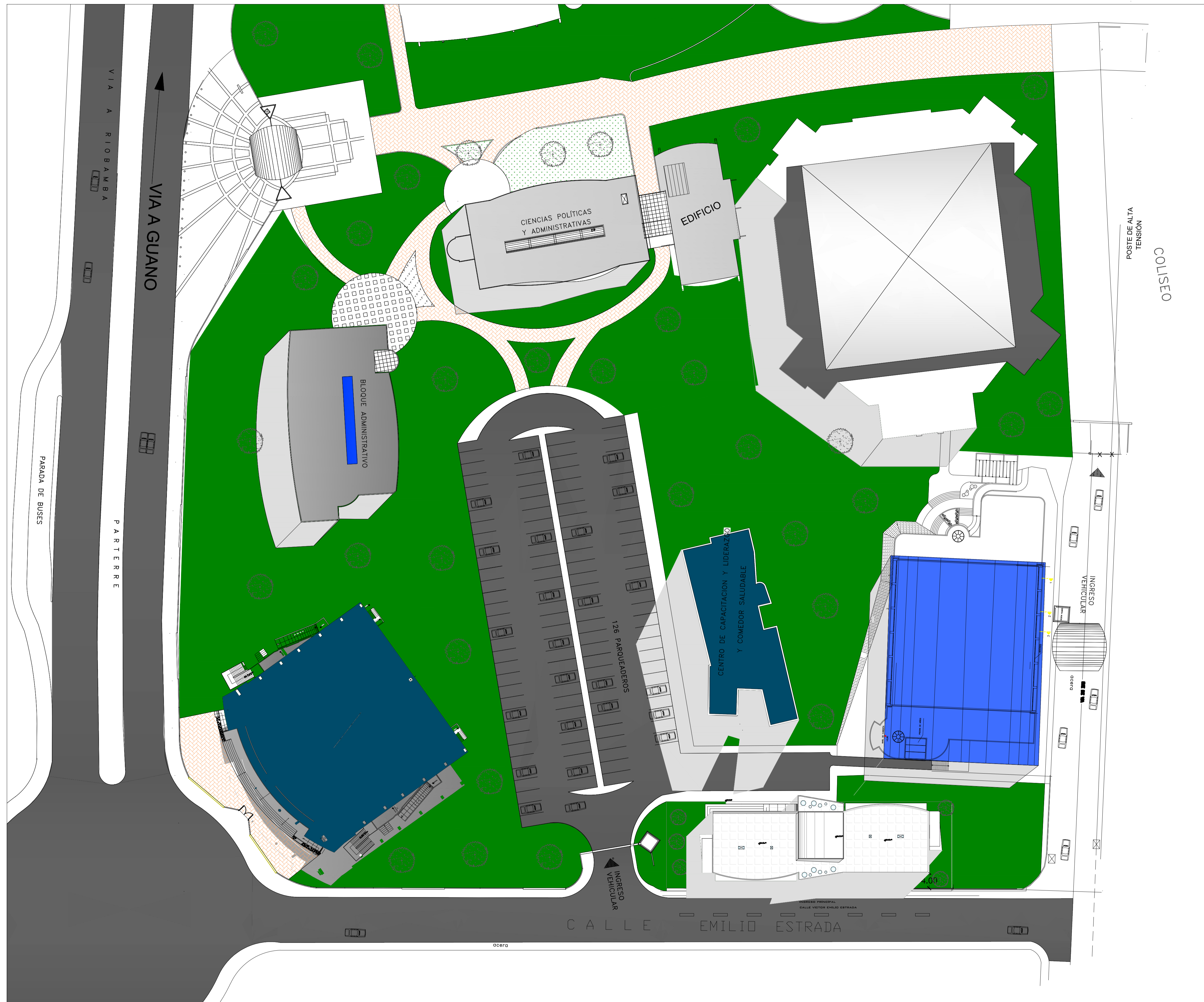
IMPLANTACIÓN GENERAL ESC 1:400
