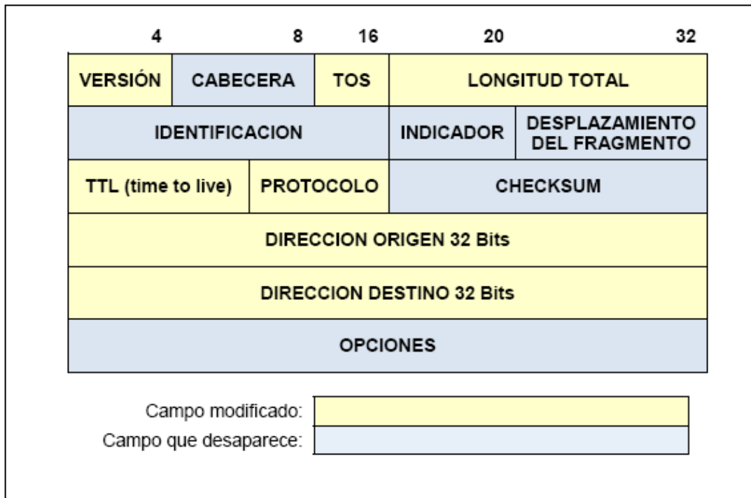
FIGURA 2.1 FORMATO DE LA CABECERA DEL PROTOCOLO IPv4 5
