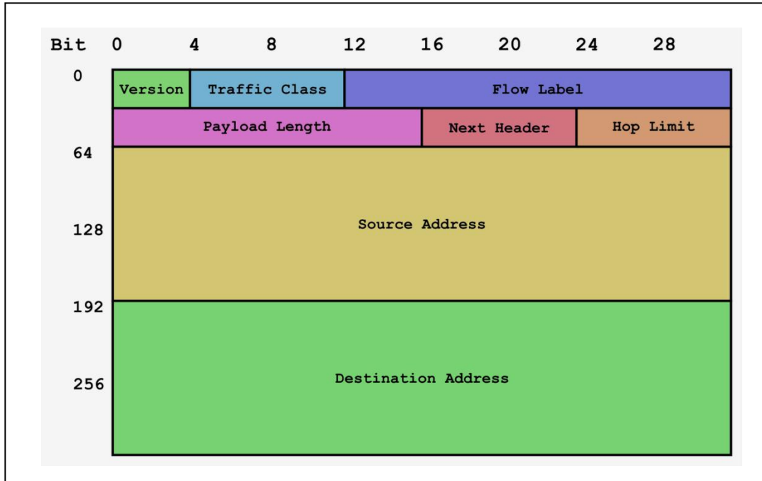
FIGURA 2.5. CABECERA IPV6 9
