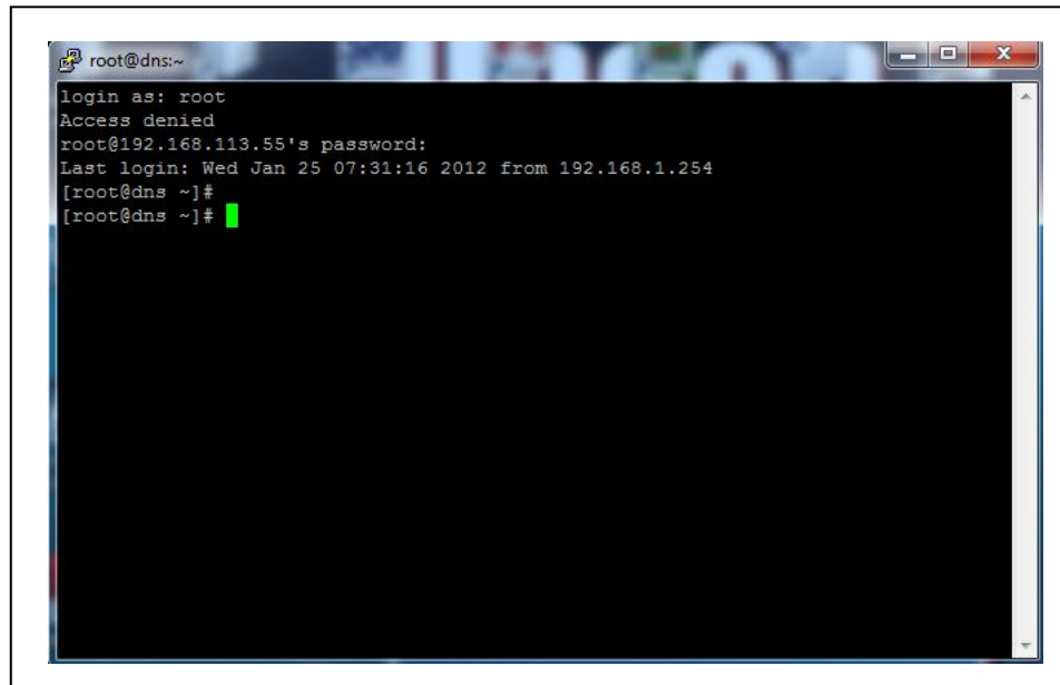
FIGURA 4.7 SERVIDOR DNS
