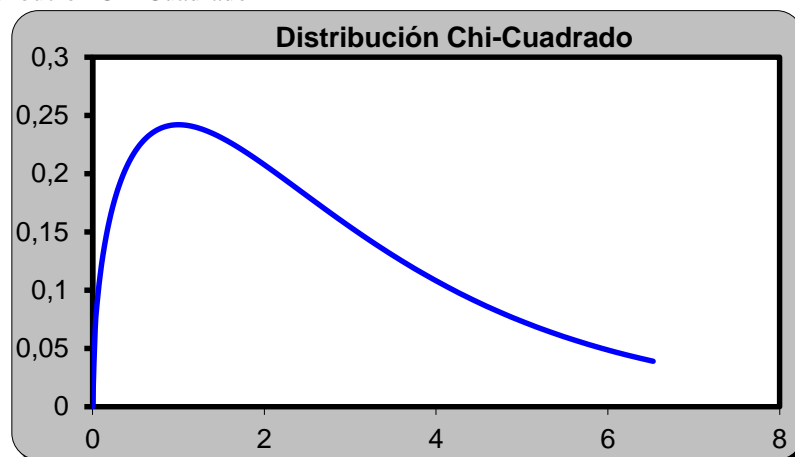
Gráfico 20. Distribución Chi-Cuadrado
